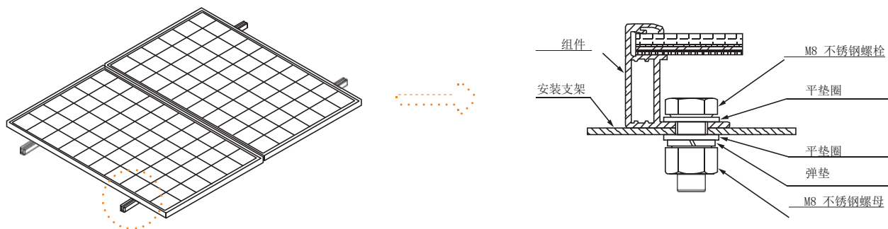
图 3 螺栓孔安装
