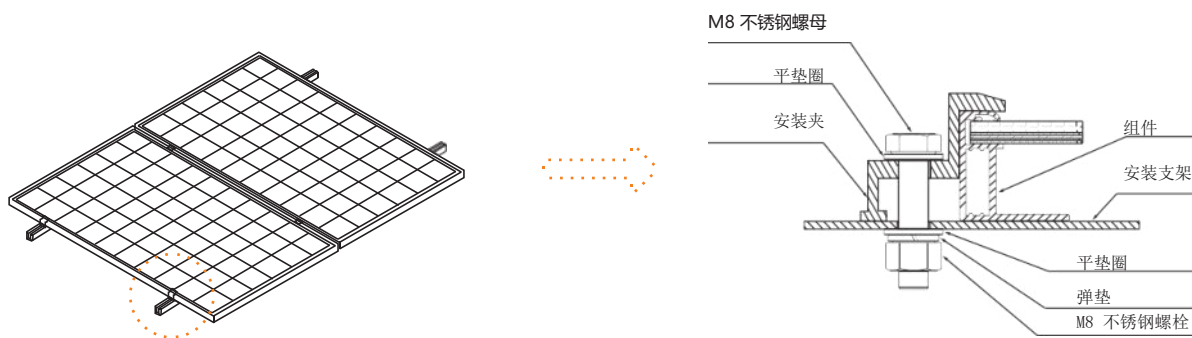
图 4 压块安装
